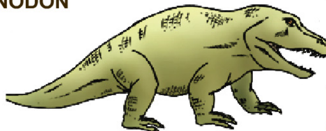
ERYTHROSUCHUS
